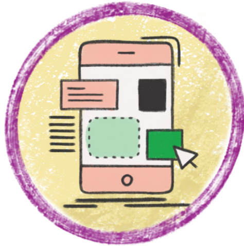
UX/UI
