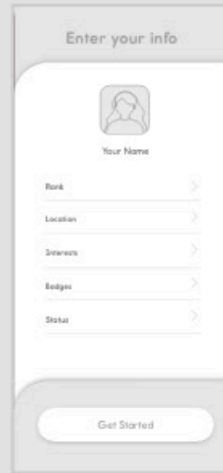
iPhone X/...
